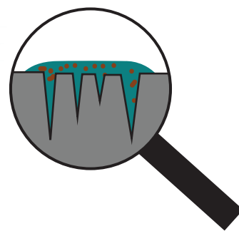
Supersmáčivý efekt
